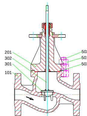
MV 5211, PV 6211 DN 15 – 50, PN 63 – 160
