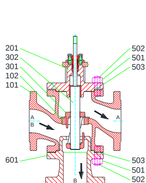
MV 5231, PV 6231 DN 100, PN 16 – 40
