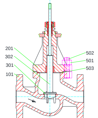
MV 5211, PV 6211 DN 65 – 100, PN 63 – 160
