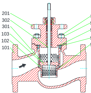
MV 5211, PV 6211 mit/ with/ avec QCS 2-stage DN 15 – 65, PN 16 – 40
