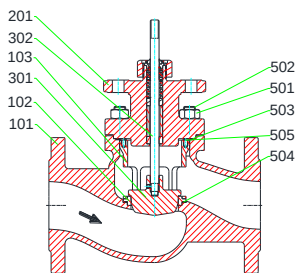
MV 5211, PV 6211 mit/ with/ avec QCS DN 15 – 65, PN 16 – 40
