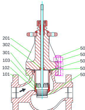
MV 5211, PV 6211 mit/ with/ avec QCS 2-stage DN 15 – 50, PN 63 – 100
