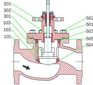
MV 5211, PV 6211 mit/ with/ avec QCS DN 80 – 100, PN 16 – 40
