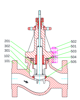
MV 5211, PV 6211 mit/ with/ avec QCS DN 65 – 100, PN 63 – 100
