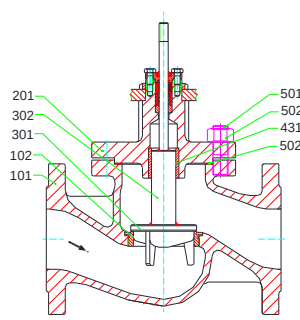
MV 5211, PV 6211 DN 80 – 100, PN 16 – 40
