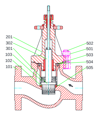
MV 5211, PV 6211 mit/ with/ avec QCS 2-stage DN 65 – 80, PN 63 – 100
