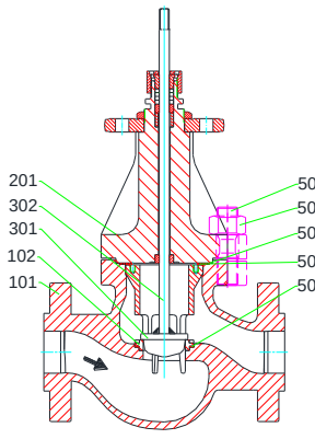
MV 5211, PV 6211 mit/ with/ avec QCS DN 15 – 50, PN 63 – 100
