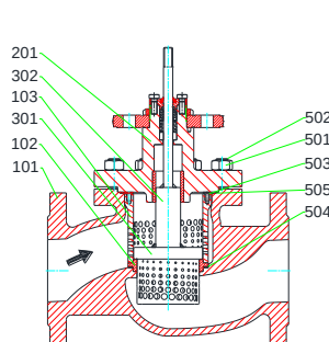
MV 5211, PV 6211 mit/ with/ avec QCS 2-stage DN 80 – 100, PN 16 – 40
