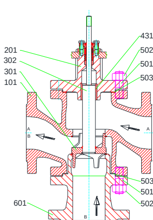
MV 5221, PV 6221 DN 100, PN 16 – 40
