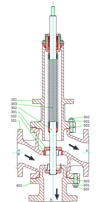
MV 5434, PV 6434 DN 80 – 300, PN 16 – 25
