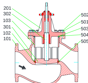
MV 54112, PV 64112 2 mit/ with/ avec QCS DN 250 – 300 2 , PN 16 – 40
