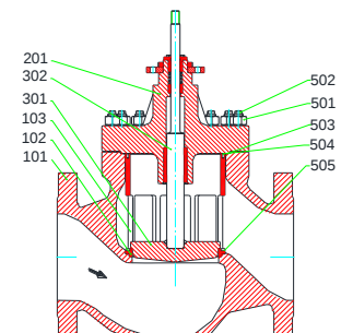
MV 54112, PV 64112 2 mit/ with/ avec QCS DN 250 – 300 2 , PN 63 – 100
